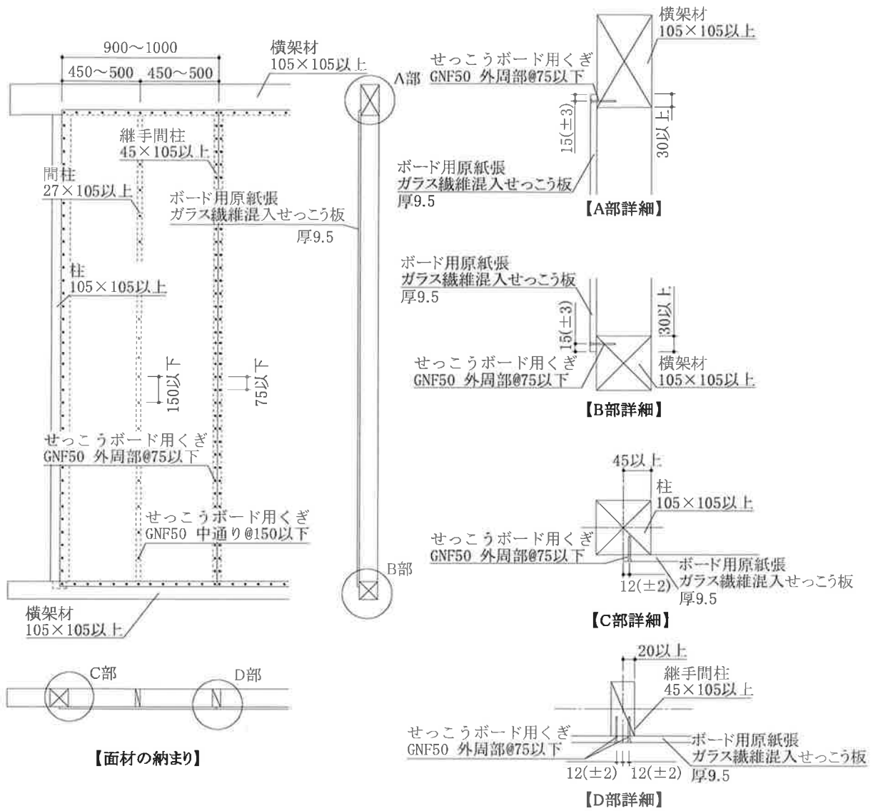
図7 施工図：1枚張りの場合 (寸法単位：mm)
