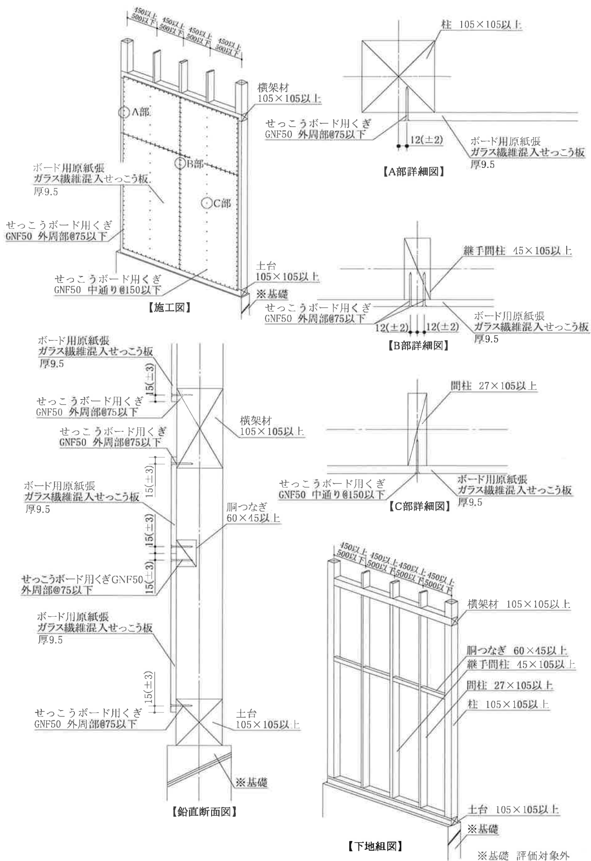
図4 施工詳細図：縦継ぎ張りの場合 (寸法単位：mm)
